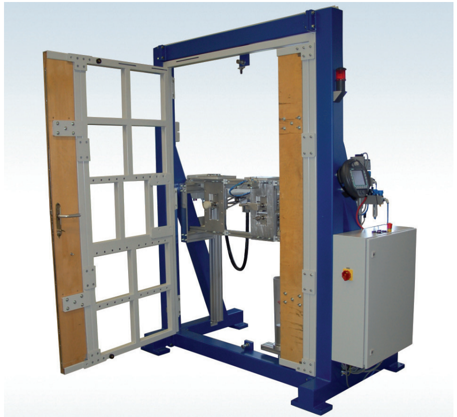
automatischer Prüfstand für Türen
